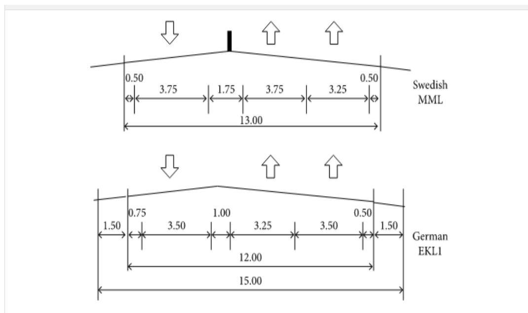
Рисунок 1 – Поперечные профили международных автомобильных дорог
